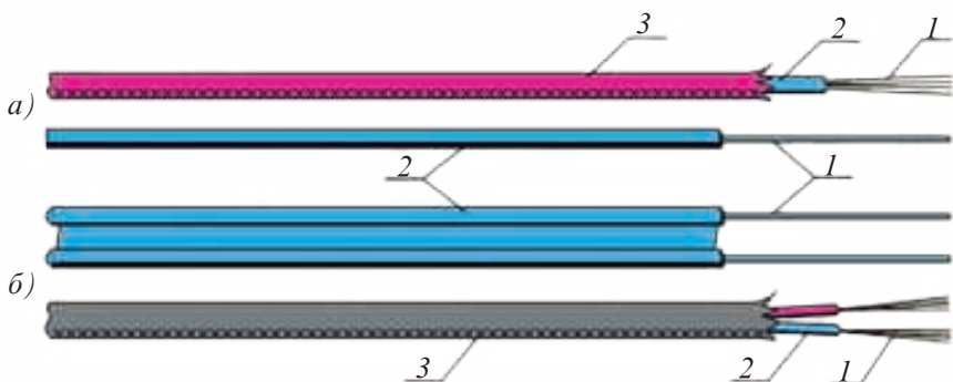
Расми 158. Симҳо (ноқилҳо) (а) ва (б): 1 - ноқили барқгузарон; 2 - изолятсия; 3 - парда.
