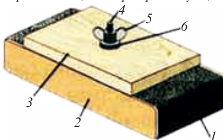
Расми 67. Кундачаи суфтакунӣ: 1 – коғзи сунбод; 2 – асос; 3 – зеҳи фишурдашаванда; 4 – винт; 5 – гайкаи фишурдашаванда; 6 – шайба
