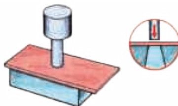
Расми 125. Тарзи сӯрохкунии механикӣ. Як ё якчанд тунукаро ба матритсаи як ё якчанд сӯрохи-дошта мегуздоранд.
