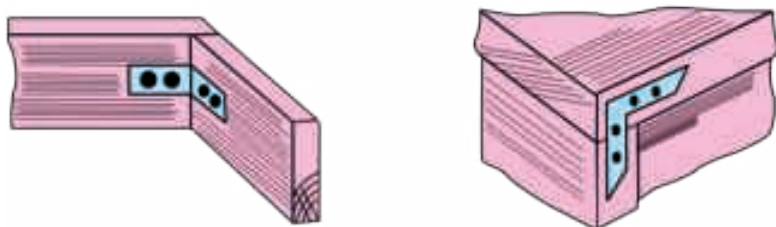
Расми 151. Таъмири кунҷҳои меҳел бо масолеҳи металлӣ.
