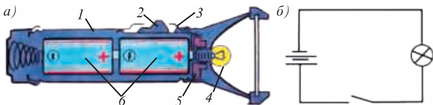
Расми 160. Сохти ҷароғи дастӣ (а) ва схемаи барқии он (б): 1 - ба- дана; 2 - даргиронанда ва хомӯшкунанда; 3 - иттисоли даргиронанда ва хомӯшкунанда; 4 - ҷароғ; 5 - изолятор; 6 - батареяҳо.
