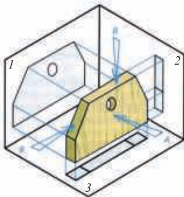
Расми 19. Намуди ҷузъҳои “девор” бо тарафҳои гуногун. А, Б, В – самтҳои биниш.
