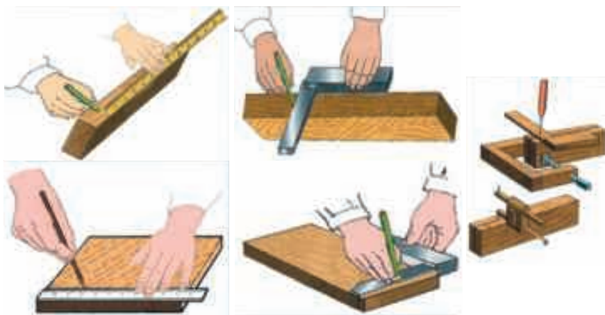
Расми 25 а. Аломатгузориҳои деталҳои росткунҷашакл: а – андозагирии хатҳои мувозӣ ва амудӣ ба воситаи хаткашак; б – сабти хатҳои мувозӣ ва амудӣ ба воситаи гул; в – андозагирии бари ашӣ сохтанишаванда аз канораи он, яъне А; г – гузаронидани хатҳои мувозӣ ба канораҳои А; д – аломатгузорӣ бо асбоби рейсмус.
