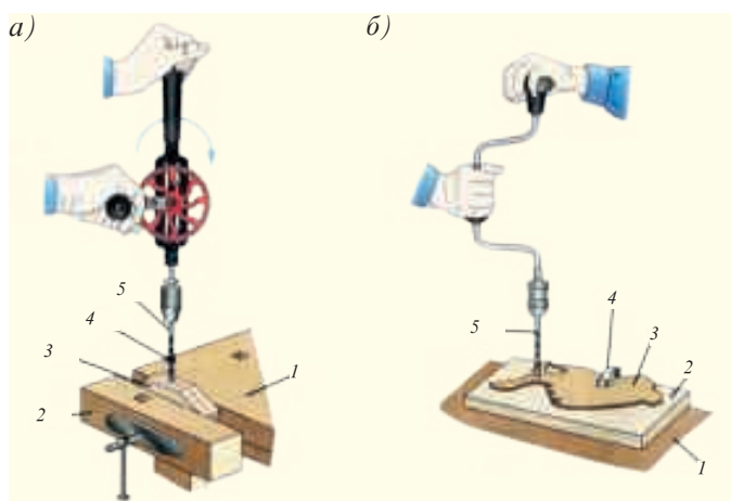
Расми 46. а - Пармакунӣ дар гирои қафои мизи дуредгарӣ: 1 – сарпӯши мизи дуредгарӣ; 2 – гирои мизи дуредгарӣ; 3 – масолеҳ; 4 – маҳдудкунанда; 5 – парма. б - Пармакунӣ бо шутургардан дар гирои қафои мизи дуредгарӣ: 1 – рӯи мизи дуредгарӣ; 2 – зертахта; 3 – масолеҳ; 4 – фишордеҳ; 5 – парма.
