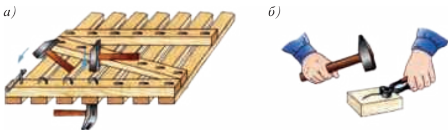
Расми 52. а – қаткунӣ ва зада даровардани қисми баромадаи мех (дар мисоли панҷараи зерӣ пой); б – рост кардани мехҳои қатшуда дар болои чортарош.
