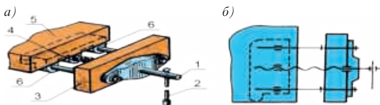
Расми 79. Ғирои винтии мизӣ дуредгарӣ (а) ва нақшаи кинематикии он (б): 1 - винти ҳаракаткунанда; 2 - даста; 3 - тахтачаи ғиро; 4 - гайка; 5 - сарпӯши миз; 6 - таъягоҳ.
