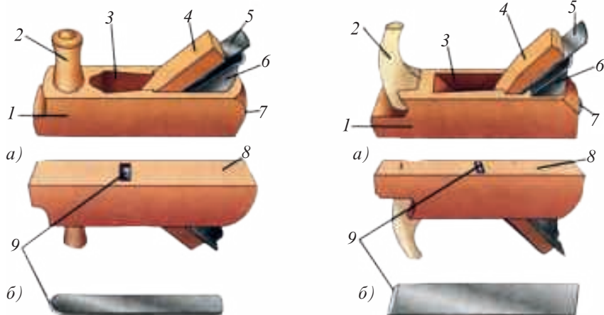
Расми 40. а - Досранда: 1 – тана; 2 – даста; 3- лона; 4 –фона; 5 –тега; 6 – тақя; 7 – ҷӯбпунба; 8 – зер; 9 – тега. б – Рандаи одӣ: 1 – тана; 2 – даста; 3 – лона; 4 –фона; 5 –тега; 6 – тақя; 7 – ҷӯбпунба; 8 – зер; 9 – тега.
