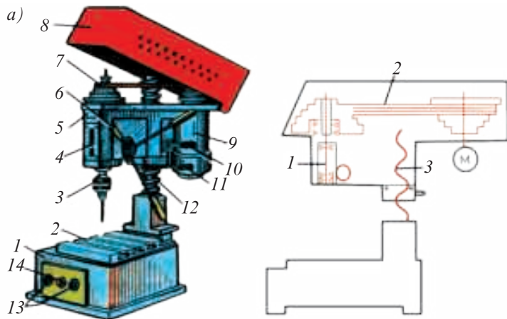
Расми 129. Дастгоҳи пармакунӣ: а - сохти умумӣ; 1 - асос; 2 - мизи корӣ; 3 - патрон; 4 - шкалаи танзими чуқурии пармакунӣ; 5 - гирои шпинделӣ; 6 - дастак; 7 - ҳаракатгузаронӣ бо тасма; 8 - рӯйкаши муҳофизатӣ; 9 - муҳаррики барқӣ; 10 - дастаи танзими гирои шпинделӣ; 11 - дастаи ба поён ҳаракатдиҳандаи гирои шпинделӣ; 12 - колонна; 13 - тугмачаҳои баҳаракатдорӣ; 14 - тугмачаи "Ист"; б - схемаи кинематикӣ 1 - ҳаракатдиҳандаи рейкагӣ; 2 - ҳаракатдиҳандаи тасмагӣ; 3 - ҳаракатдиҳандаи винтӣ.
