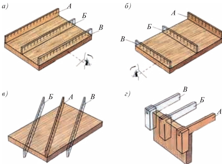
Расми 42. Санҷидани ростхаттии сатҳи масолеҳ (а – в) ва мувозӣ будани паҳлу нисбати сатҳ (г).
