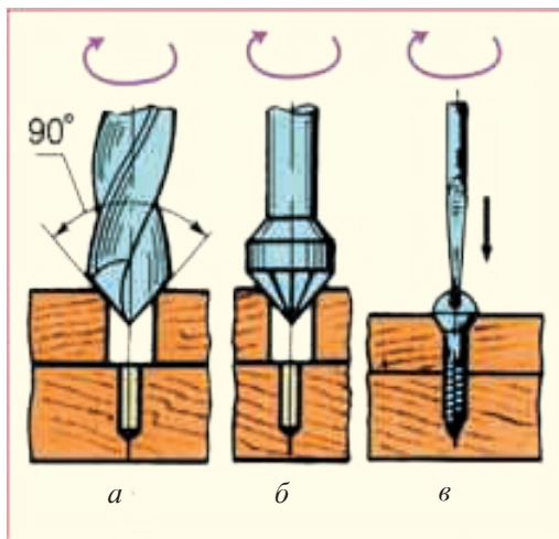
Расми 54. Тайёр кардани ҷойи сараки рахпеч: а - бо парма; б - бо зенковка; в - тоб додани рахпеч бо мурваттоб.
