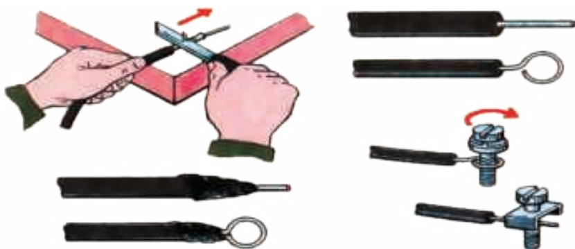
Расми 174. Пайиҳаҳои ҳалқакунии ва пайвастикунии симҳо
