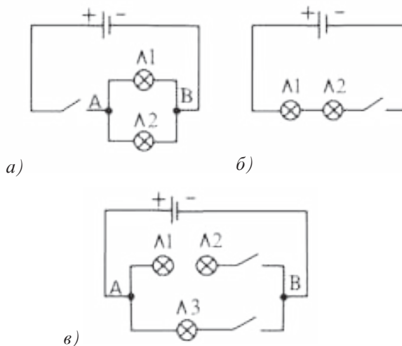
Расми 161. Тарзҳои гуногуни пайваستкунии ҷароғи барқӣ ба манбаи барқ: а - мувозӣ; б - пайиҳам; в - омехта.
