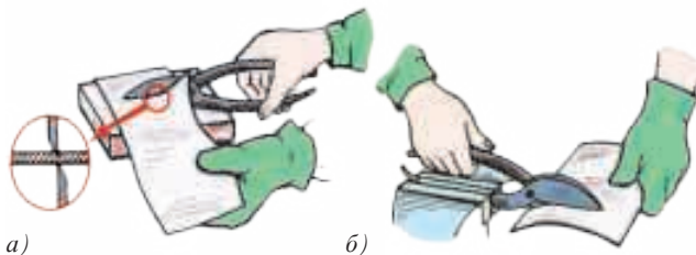
Расми 108. Буридани тунука бо қайчӣ: а – дар рӯйи миз ва б – дар исканҷ.
