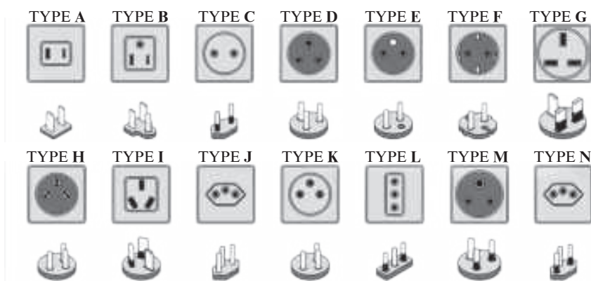
Расми 169. Навъҳои барқбун ва барқчангҳо дар ҷаҳон
