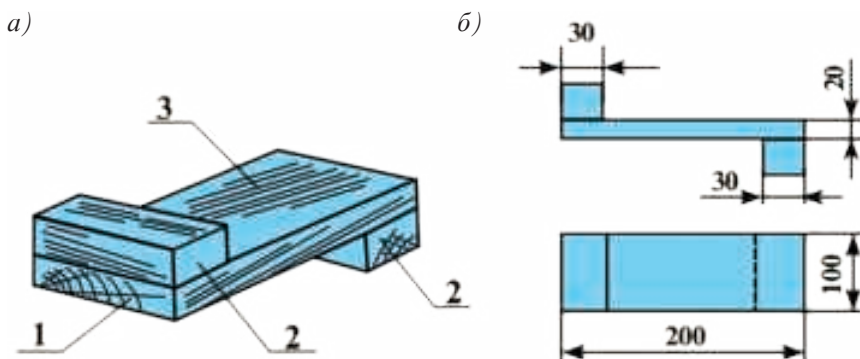
Расми 195. Олоти арракунӣ: а - расми техникӣ (1 - асос; 2 - такиягоҳ; 3 - меҳи 3x4 мм) ва б - нақша.
