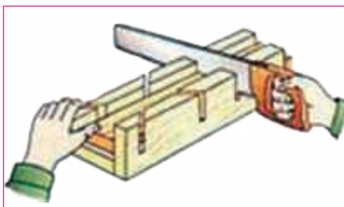
Расми 35. Арракунии бо ёрии стусло: 1- асос; 2 - девораҳо; 3 – тахтамасолеҳ, 4 - арра.
