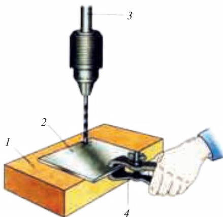
Расми 132. Сӯрохкунии тунука дар болои зертахта: 1 – зертахта; 2 – тунука; 3 – шпиндели дастгоҳ; 4 – исканҷи дастӣ
