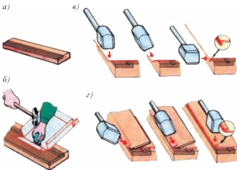
Расми 118. Қаткунии тунукаҳои дароз: а - асбоби қаткунӣ, б, в, з - тарзҳои қаткунӣ.
