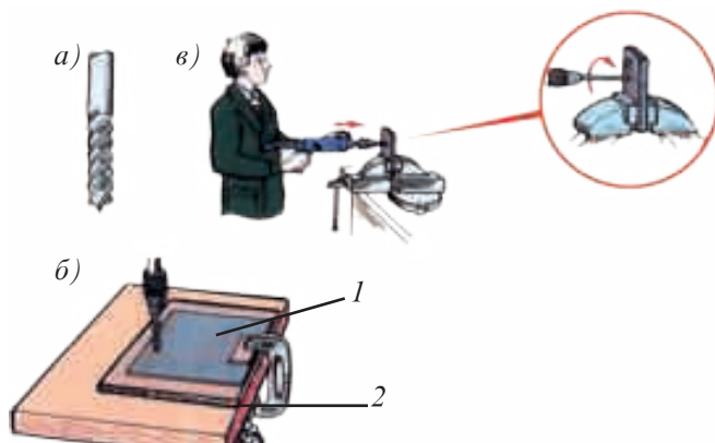
Расми 127. Парма барои сӯрох кардани тунука (а) ва тарзҳои пармакунӣ (б, в): 1 - маҳсулоти сӯрохшаванда, 2 - тахтача.
