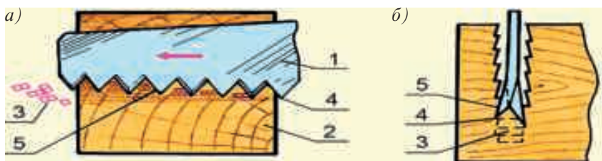
Расми 32. Буриши кўндаланг: а - намуд аз паҳлуи арра; б - намуд аз буриши: 1 - арра; 2 - масолех; 3 - аррамайда; 4 - нўги дандони арра; 5 – тегаи бурандаи дандони арра.
