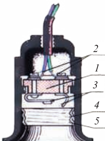
Расми 165. Патрони овезаи лампа: 1 – дила; 2 – гироҳои винтӣ; 3 – иттисолҳои пружинӣ; 4 – рахпеч; 5 – бадана.
