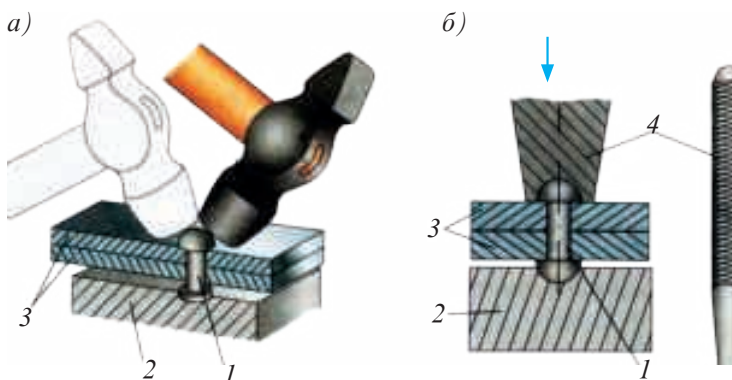
Расми 140. Ба шакли муайян даровардани сараки парчинмех: а – бо ёри болға; б – фишорқолаб; 1 – парчинмех; 2 – таёя; 3 – ҷузъҳо; 4 – фишорқолаб.
