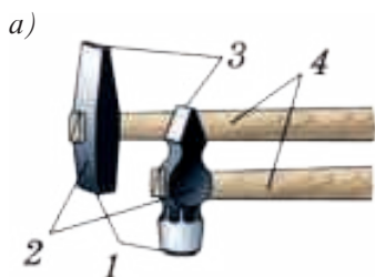
Расми 90. Асбобҳои зарбазананда: а – болғаи челонгарӣ: 1 – зарба-наки доирашакл ва чоркунҷашакл; 2 – сарак; 3 – нӯг; 4 – даста; б – болғаи чӯбин: 1 – сарак; 2 – даста.
