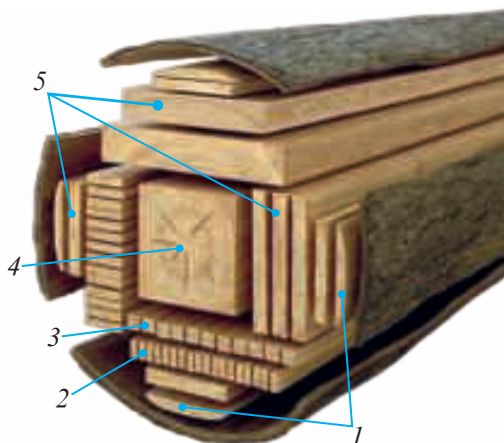
Расми 10. Навъҳои масолеҳи чӯбу тахта аз гӯлачӯб: 1 – тахтаи тахта; 2 – тахтаи буридашуда; 3 – чӯби чортарош; 4 – чӯби чортарош; 5 – тахтаи буридашуда.
