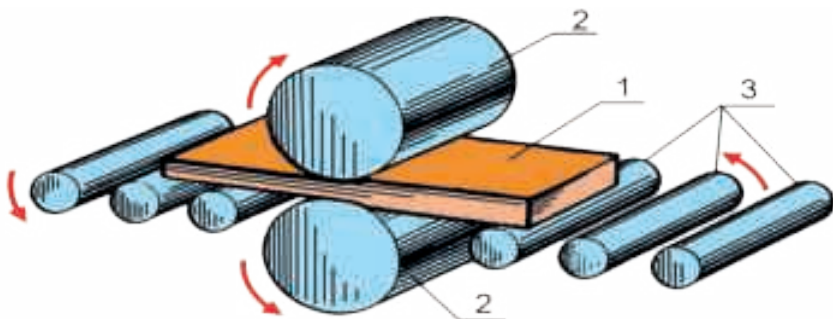
Расми 88. Схемаи ҳосил кардани тунука: 1 - моли хом ё худ масолеҳ; 2 - навардҳо; 3 - гилдиракҳо.
