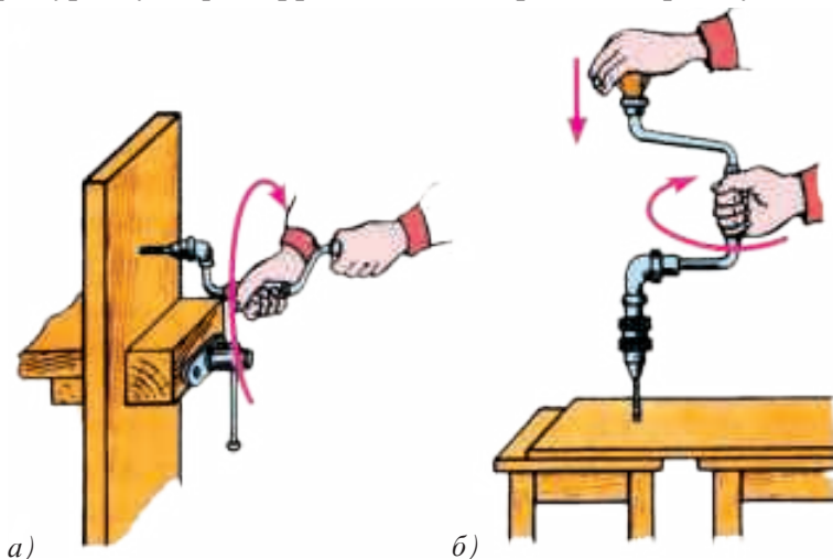
Расми 47. Тарзҳои пармакунӣ: а - дар гирои мизи дуредгарӣ; б - дар рӯйи сатҳ.
