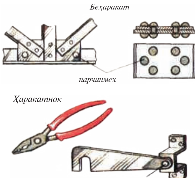
Расми 138. Намудҳои пайванди парчинмех.
