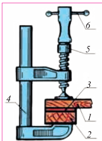
Расми 60. Фишордеҳ: 1, 2- деталҳои ширишиаванда; 3 - шириш; 4 - танаи фишордеҳ; 5 - печи фишордеҳ; 6 - дастаи фишордеҳ.
