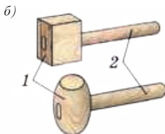
Расми 90. Асбобҳои зарбазананда: а – болғаи челонгарӣ: 1 – зарба-наки доирашакл ва чоркунҷашакл; 2 – сарак; 3 – нӯг; 4 – даста; б – болғаи чӯбин: 1 – сарак; 2 – даста.
