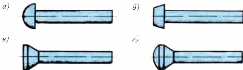
Расми 136. Навъҳои парчинкунӣ бо парчинҳои саракҳои гуногундошта.
