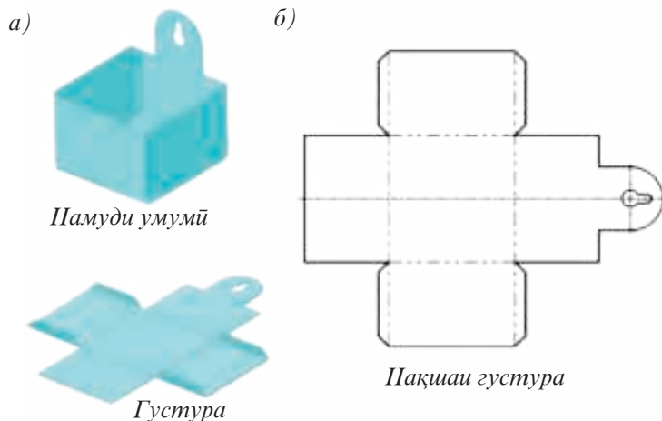
Расми 95. Маҳсулоти ҳаҷмдор аз тунука: а - расм; б - нақшаи густара
