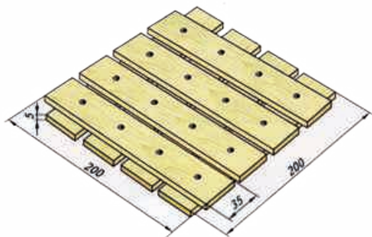
Расми 199. Таҳмон барои зарфҳои гарм.
