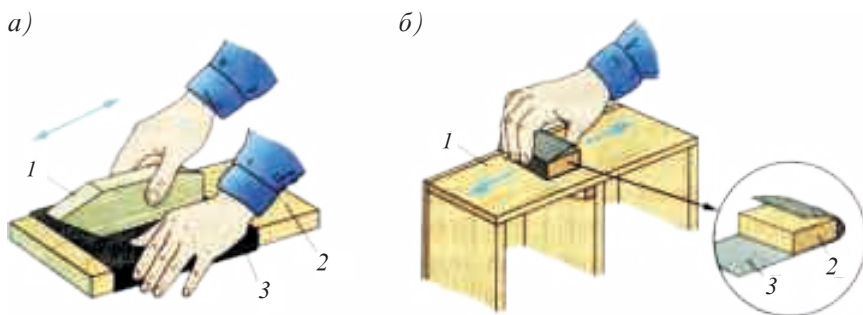
Расми 66. а – суфтакунии ҷузъҳо: 1 – ҷузъ; 2 – зертахта; 3 – коғзи сунбод б – суфтакунии сатҳи калон бо коғзи сунбод: 1 – сатҳи коркардишаванда; 2 – чортароши ҷӯбӣ; 3 – коғзи сунбод.
