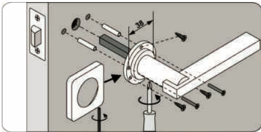
Расми 152. Нақшаи насби дастии дар.
