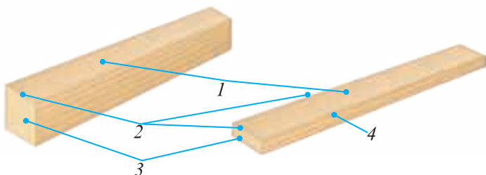
Расми 13. Унсурҳои масолеҳи чӯбу тахта: 1 – рӯя; 2 – қира; 3 – нӯг; 4 – зеҳ (рах).
