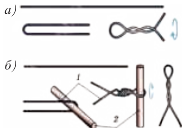
Расми 104. Тарзҳои тоб додани сим: а – бе ёрии тир; б – бо ёрии тир: 1 – масолеҳ аз сим; 2 – тир (олоти дастгоҳҳои металлбурӣ барои нигоҳ доштани асбобу маснуот).
