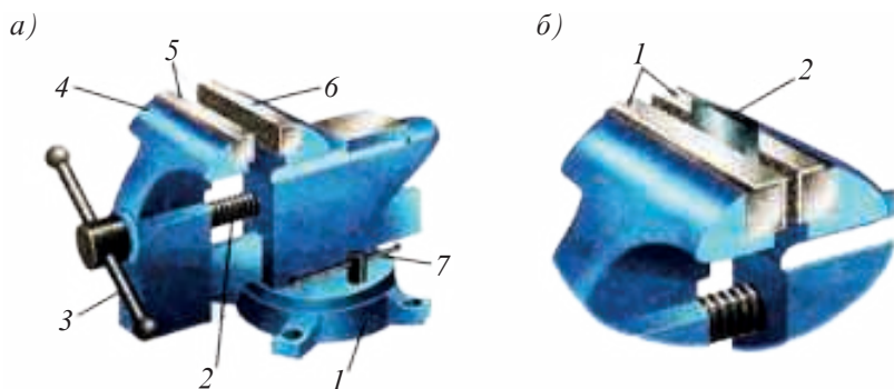
Расми 85. а - исканҷҳои челонгарӣ: 1 - лавҳаи таъягоҳӣ; 2 - винти ҳаракаткунанда; 3 - даста; 4 - лаби беҳаракат; 5 - зеҳи фишордиҳӣ; 6 - лаби ҳаракаткунанда; 7 - дастаи мустаҳкамкунӣ. б - мустаҳкамкунии масолеҳи металли мулоим дар исканҷ: 1 - лабаҳо; 2 - масолеҳ.
