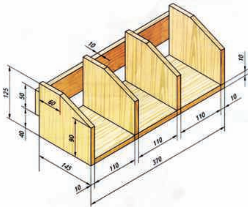
Расми 198. Раф барои тубакҳои гул.
