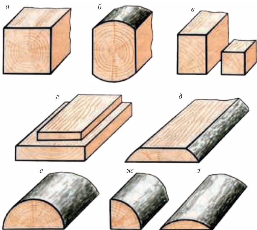
Расми 12. Маҳсулоти гуногуни чӯбӣ: а - чӯби чортарош, б - чӯби дутарош; в - чӯби чортароши хурд; г - тахтаҳои буридашуда; д - тахтаҳои буриданашуда; е - лавҳаҳо; ж - чорякчӯб; з - пуштатахта.
