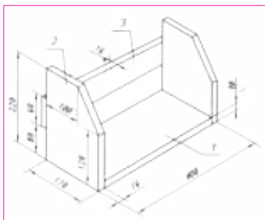
Расми 56. Рафи рӯйимизӣ барои китобҳо: 1 – асос; 2 – девори паҳлӯӣ; 3 – зеҳи тахтагӣ.
