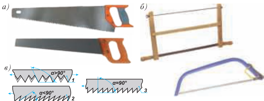
Расми 31. Навъҳои арра: а - дастарраҳо; б - камонарраҳо; в - дандонаи арраҳо. 1 - дандонаҳо барои арракунии кӯндаланг; 2 - дандонаҳо барои арракунии ба дарозӣ, барқад; 3 - дандонаҳо барои арракунии гуногун.
