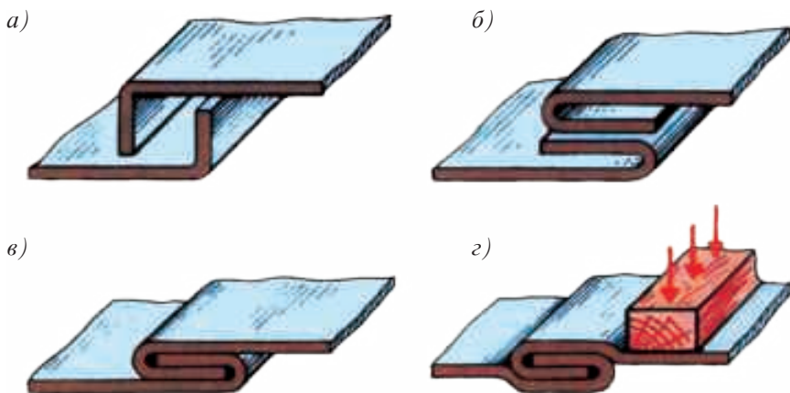
Расми 135. Пайдарпайии ҳосил кардани қатпайванд.
