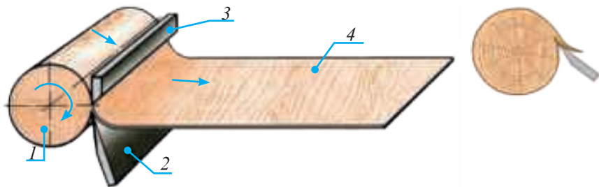
Расми 15. Схемаи буридани тахтаварақ барои фанер: 1 - гӯлачӯб; 2 - теғ; 3 - ҷафсақ; 4 - варақаҳои шпон.
