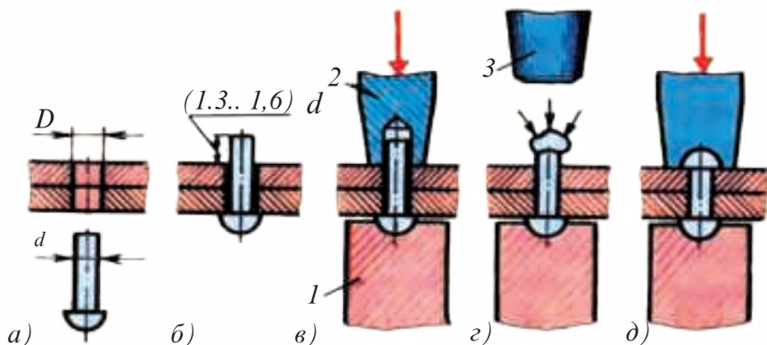
Расми 137. Марҳалаҳои пайвасткунӣ ба воситаи парчин: а — сӯрохкунӣ; б - ҷойгир кардани парчин; в - ҷойгир кардани маҳсулоти парчиншаванда; г - парчин кардани сарак; д - шаклдиҳии парчини сарак (1 - кашии додан; 2 - дошта истодан; 3 - болга; 4 - фишурдан).
