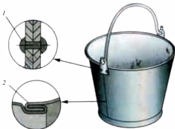
Расми 139. Намунаи пайвасти ҷузъҳо аз тунука: 1 – пайвасти парчин-мех; 2 – ҷаттайванд.
