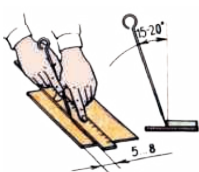
Расми 100. Гузаронидани хатти намуна.
