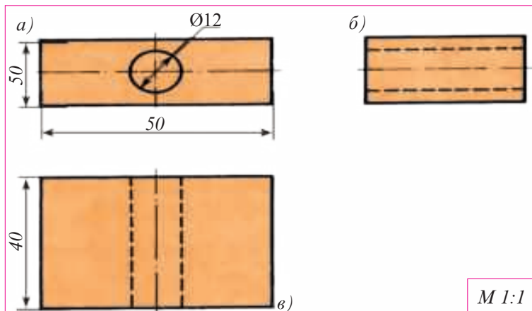
Расми 18. Нақшаи ҷузъ-детал: а - намуди асосӣ; б - намуд аз паҳлу; в - намуд аз боло.
