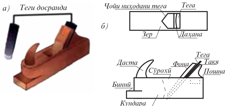
Расми 39. Досранда: а – намуди умумӣ; б – намуд аз поён; в – намуд аз паҳлу.
