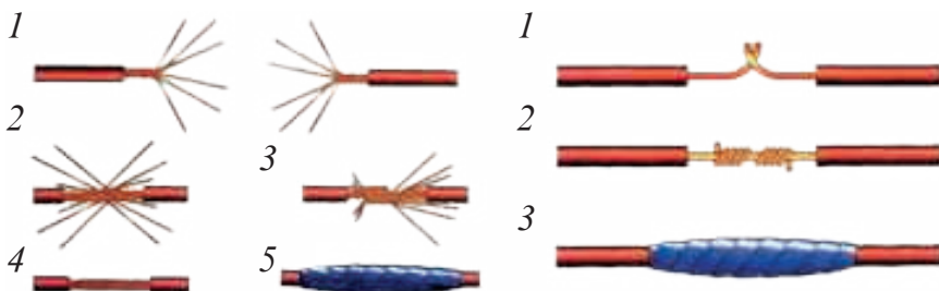
Расми 173. Тармими ноқили қатъшуда.
