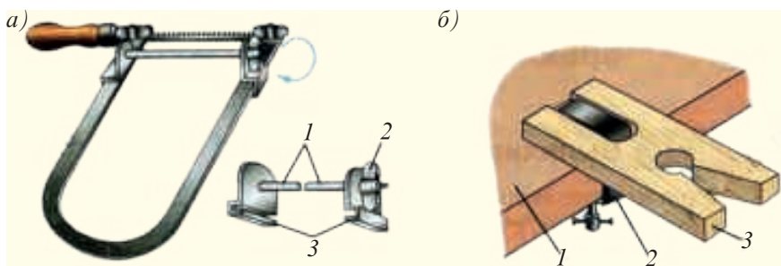
Расми 69. а – маҳкамқунии симарра: 1 – итилкаи рахпечӣ; 2 – чайка; 3 – кашолақунак. б - таҷҳизот барои фишурдани канораҳои ҷавкот
