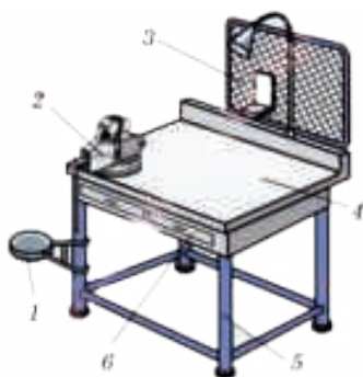
Расми 82. Мизи челонгарӣ: 1 - ҷойи нишаст; 2 - ис- канҷ; 3 - тӯри муҳофизатӣ; 4 - сарпӯш; 5 - ноя; 6 - қуттӣ.
