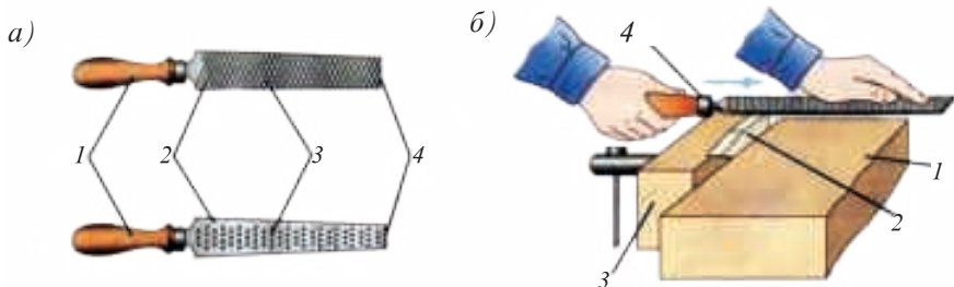
Расми 65. Навъҳои сӯхон: а – рахдор; б – нуқтавӣ: 1 – даста; 2 – қисми корӣ; 3 – пайкан; 4 – нӯг. б – тоза кардани ҷузъ бо сӯхон: 1 – сарпӯши мизи дуредгарӣ; 2 – ҷузъи коркардишаванда; 3 – гирои пеши мизи дуредгарӣ; 4 – сӯхон.
