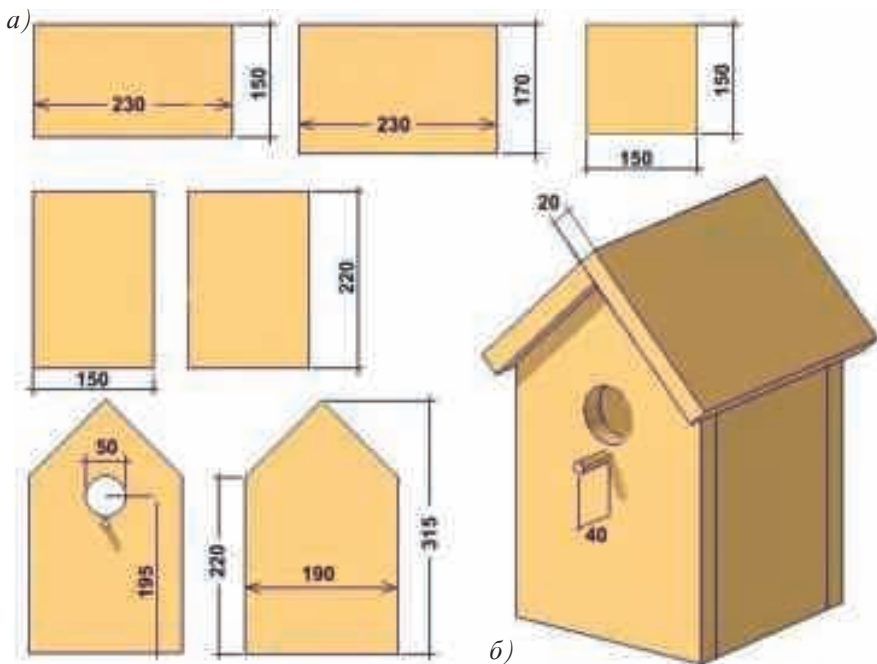
Расми 23. Нақшаҳои ҷузъиёти хонача барои паранда (а), расми техникийи он (б).
