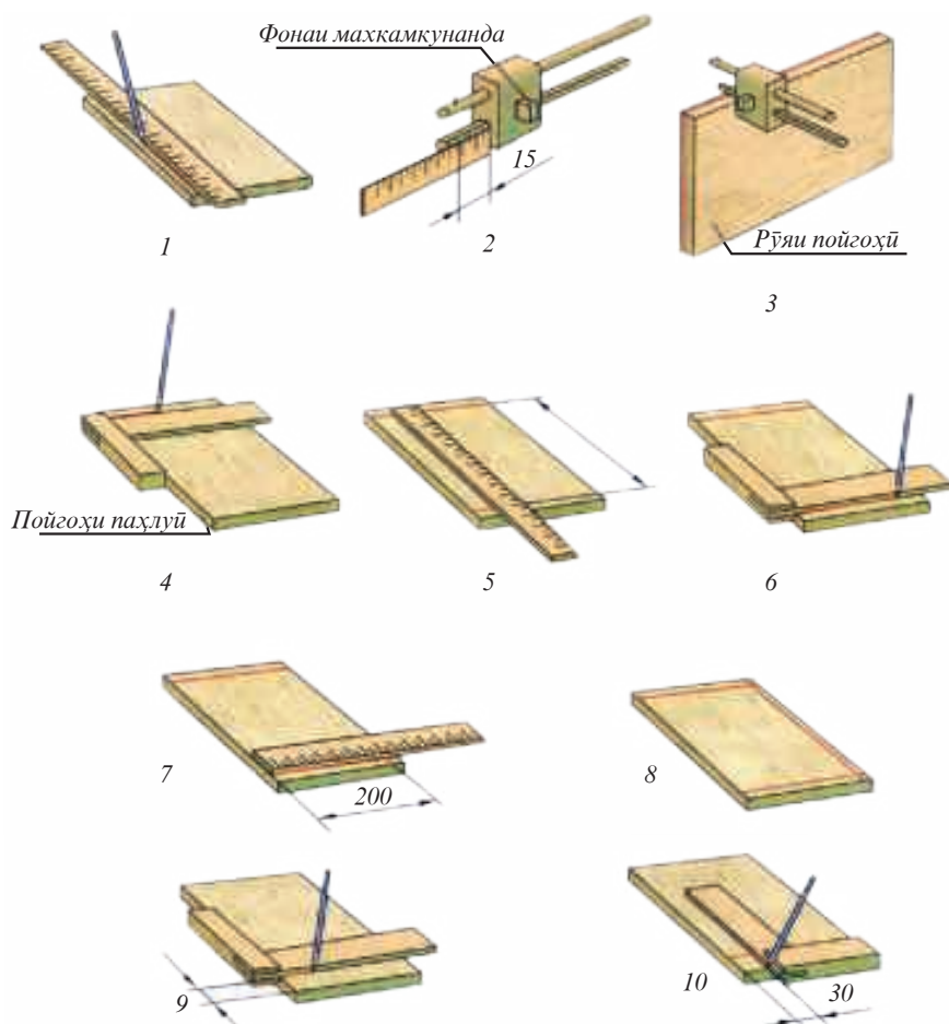
Расми 28. Пайдарҳамии аломатгузори масолеҳи ҷӯбу тахта.
