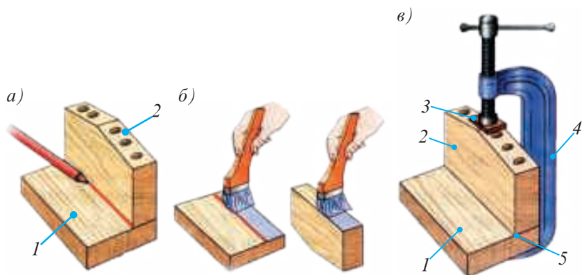
Расми 61. Пайваستкунии ҷузъҳо бо шириш: а – нишонагузориҳои ҳудуди ширишкунӣ; б – молидани шириш ба ҷузъҳо; в – маҳкам кардани ҷузъҳо дар исканҷа: 1 – асос; 2 – қаламдон; 3 – зермонак; 4 – исканҷа; 5 – ҷойи пайванд.
