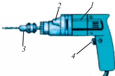
Расми 128. Пармаи барқӣ: 1 - қисми ҳаракаткунанда; 2 - қисми ҳаракатдиҳанда; 3 - қисми қорӣ, 4 - қисми идорақунӣ.
