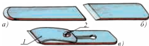
Расми 37. Тегҳо: а - теги досранда; б - рандаи одӣ; в - рандаи одӣ бо тарошашикан. 1 - тарошашикан, 2 - чархпеч.
