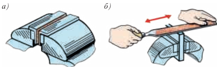
Расми 114. Тоза кардани маҳсулот ба воситаи сӯҳон: а - рӯйкаши ис- канч ва б - суфтакунии ашӯи хом бо сӯҳон.
