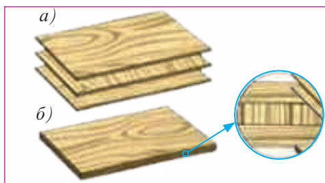
Расми 16. Тайёр кардани фанер аз варақаҳои ипон: а – ҷойгиршавии нахҳо ҳангоми пайваस्तкунии варақаҳои ипон; б – фанери ширешишуда.
