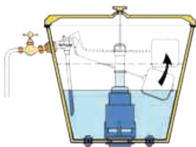
Расми 155. Сохти зарфи ташноб
