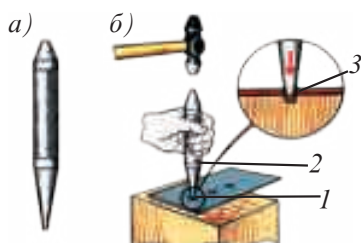
Расми 124. Сӯрох кардани металл ба воситаи сунба: а - сунба; б - раванди сӯрохкунии; 1 - ҷойи болгазани; 2 - бадана; 3 - нӯг
