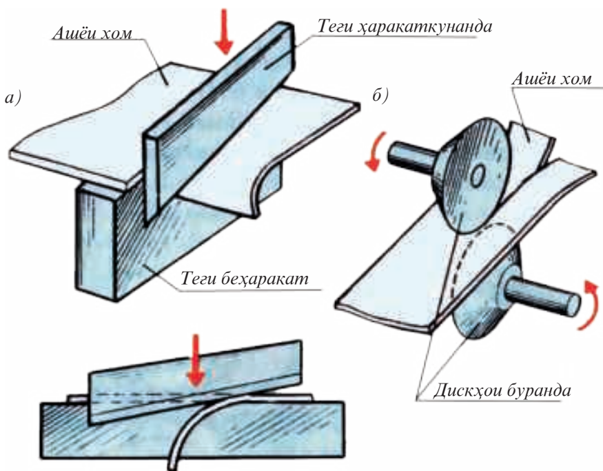
Расми 110. Буридани тунука бо қайчиҳои механикӣ: а - гилйотинӣ ва б - чархӣ.
