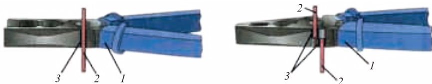
Расми 112. Буридани сим бо ёрии қисми паҳлуи дандонаи анбӯри паҳндон: 1 – анбӯри паҳндон; 2 – сим; 3 – дандонаи паҳлӯй.
