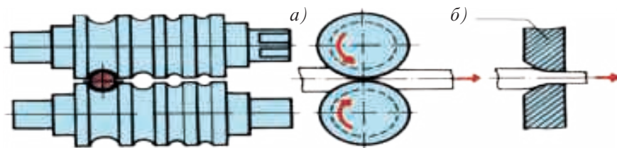
Расми 93. Схемаи ҳосил кардани сим: а - ба воситаи наварди ҷӯякдор; б - ба воситаи филер - детали сӯрохдор.
