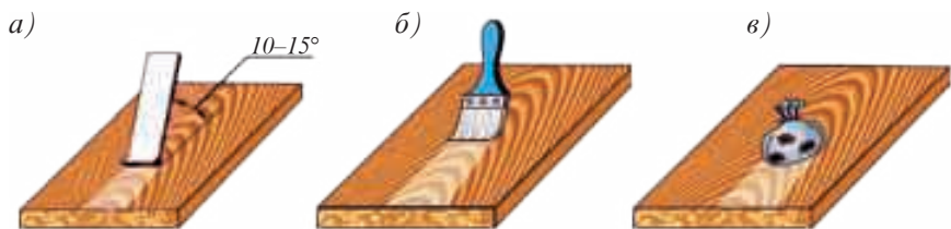
Расми 76. Ороиши чӯб: а – суфтакунӣ; б – локдихӣ бо ёри мӯқалам; в – локдихӣ бо ёри дока
