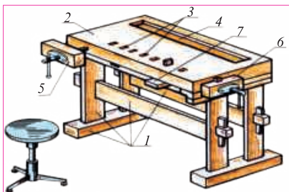
Расми 2. Мизи дуредгарӣ: 1 – асос; 2 – сарпӯш; 3 – сӯрохиҳо барои фона; 4 – нова; 5 – гирои пеш; 6 – гирои қафо; 7 – ангиштҳои ҳаракаткунанда.
