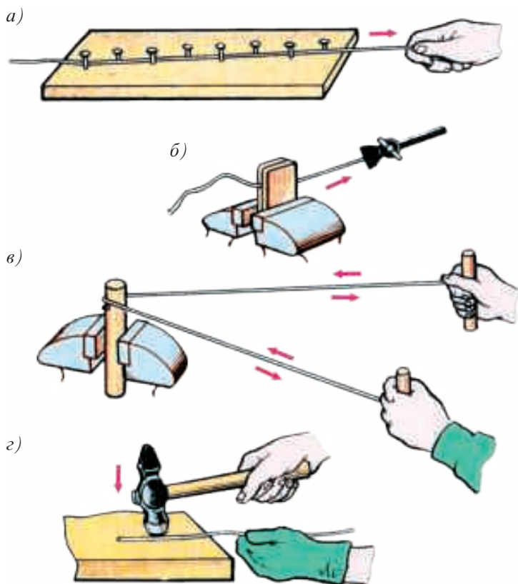
Расми 98. Рост кардани симҳо.
