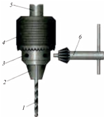
Расми 131. Патрони семуштакдори пармакунӣ: 1 – парма; 2 – муштакҳо; 3 – втулка; 4 – ҳалқа; 5 – шпиндел; 6 – калид
