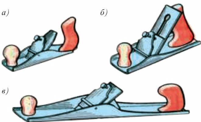
Расми 36. Навъҳои рандаҳо: а - досранда, б - рандаи одӣ, в - ҷафсранда ё дарозранда.
