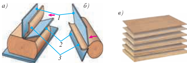
Расми 14. Масолеҳи варақагии чӯбу тахта: гирифтани як қабати шпон: а – тарошидани шпон; б – пўсткани шпон: 1 – такия; 2 – тега; 3 – шпон; в – фанера.
