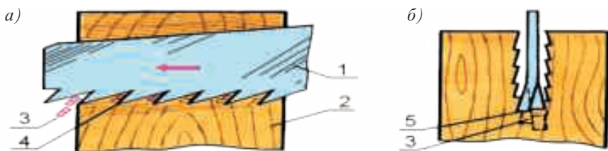
Расми 33. Буриши барқад: а – намуд аз паҳлу, б – намуди буриши арра; 1-арра, 2 – масолех, 3 – аррамайдаҳо, 4 – нўги дандона, 5 – тегаи бурандаи дандона.
