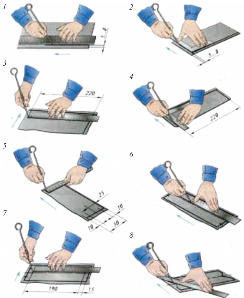
Расми 102. Пайдарҳамии аломатгузори ҷузъ аз тунука (1-8)
