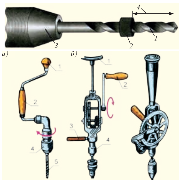
Расми 45. Асбобҳои пармакунӣ: а - шутургардан; б - парма; 1 - тақягоҳ; 2 - дастаи тобдиҳӣ; 3 - дастаи устуворгирӣ; 4 - патрон; 5 - парматег.
