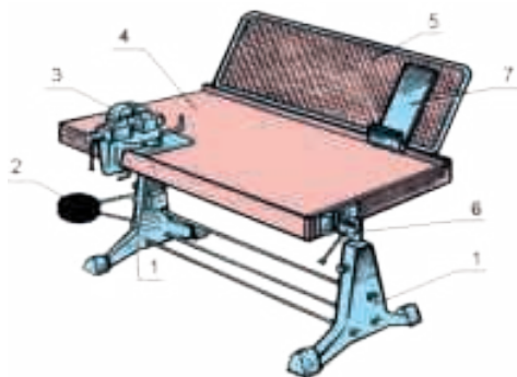
Расми 81. Мизи челонгарии универсалий: 1 - асос; 2 - ҷойи нишаст; 3 - ис- канҷи челонгарӣ; 4 - сарпӯш; 5 - симтӯри муҳофизатӣ; 6 - гирои миз; 7 - ҷойи гу- зоштани ҳуҷҷатҳои техникӣ.
