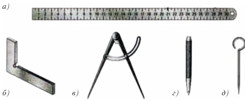
Расми 99. Асбобҳо барои аломатгузорӣ дар қорҳои челонгарӣ: а – ҷадвали металлӣ; б – гунёи челонгарӣ; в – паргори аломатгузорӣ; г – сунба; д – хаткаш.
