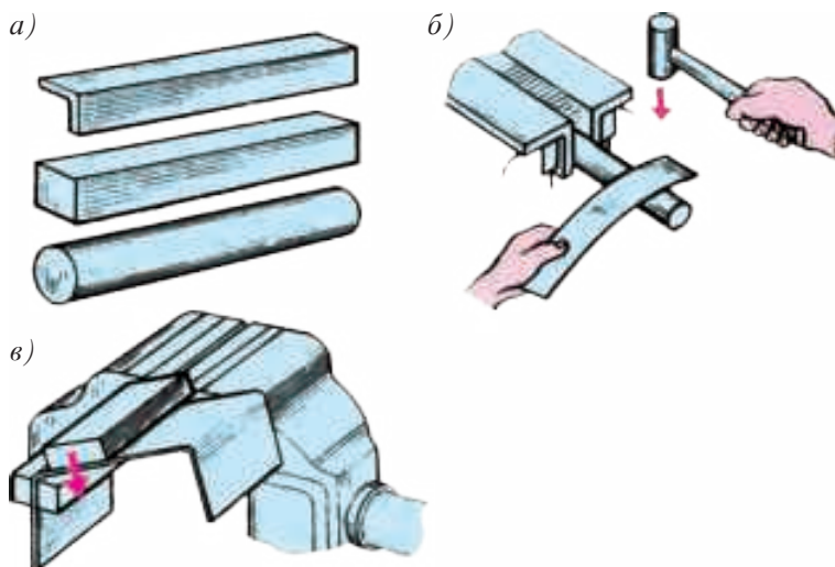
Расми 116. Қаткунии тунука ба воситаи қолабҳои филиззӣ: а - қолабҳои филиззӣ; б, в - тарзҳои қаткунии.
