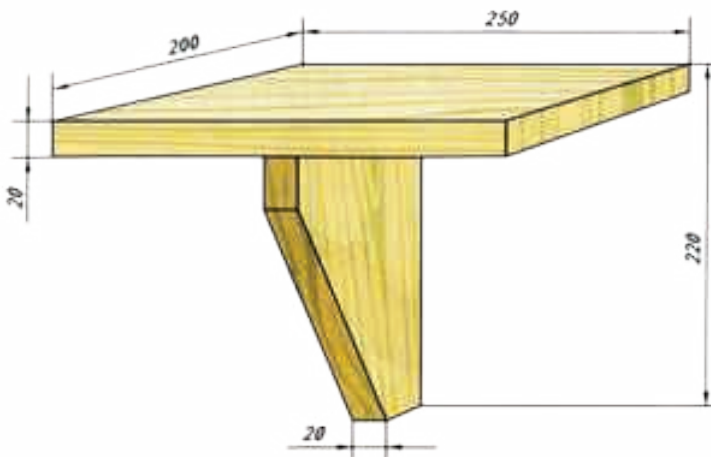
Расми 197. Рафи рӯимизӣ барои ғиттаҳо ва дискҳо.
