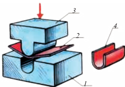
Расми 119. Қаткунӣ ба воситаи қолаб: 1 - матритса; 2 - ашӯи хом; 3 - қолаб-пуансон; 4 - маҳсулоти тайёр.
