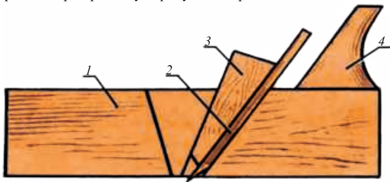
Расми 38. Сохти рандаи одӣ: 1 - асос ё тана; 2 - тег; 3 - фона; 4 - даста.
