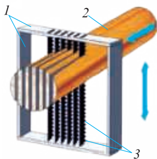
Расми 11. Дастгоҳи арракунии гӯлачӯбҳо: 1 – чортӯба; 2 – гӯлачӯб; 3 – арраҳо.
