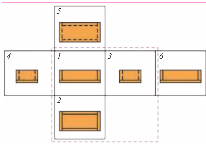
Расми 22. Шаи намуди маҳсулот. 1 - асосӣ (аз пеш); 2 - аз боло; 3 - аз чап; 4 - аз рост; 5 - аз поён; 6 - аз қафо.
